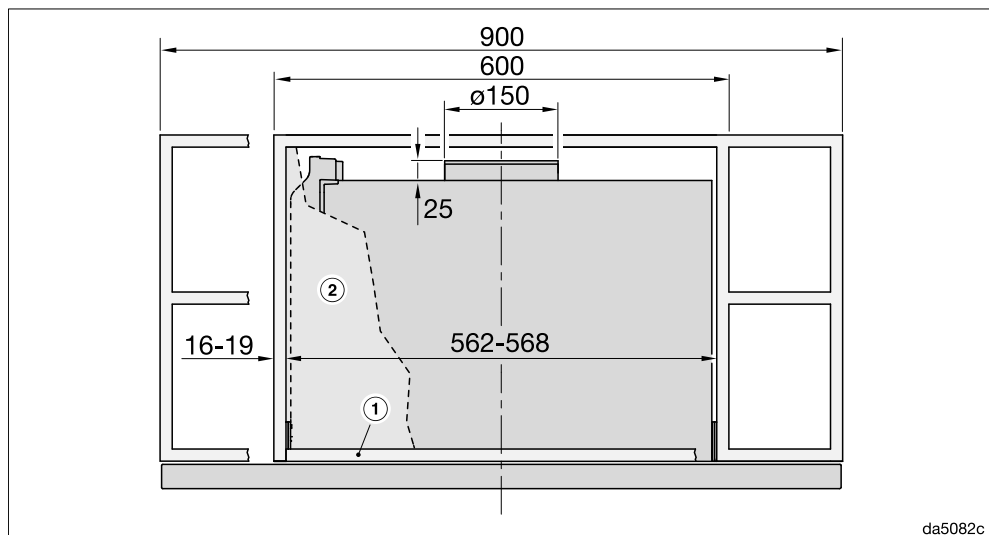
Рис. 3. DAS 4930 в шкаф шириной 600 мм или в шкаф 900 мм с боковыми отделениями
