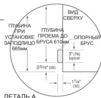
ДЕТАЛЬ А
