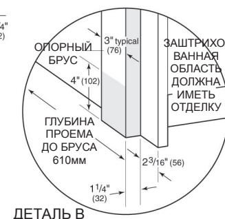
ДЕТАЛЬ В
