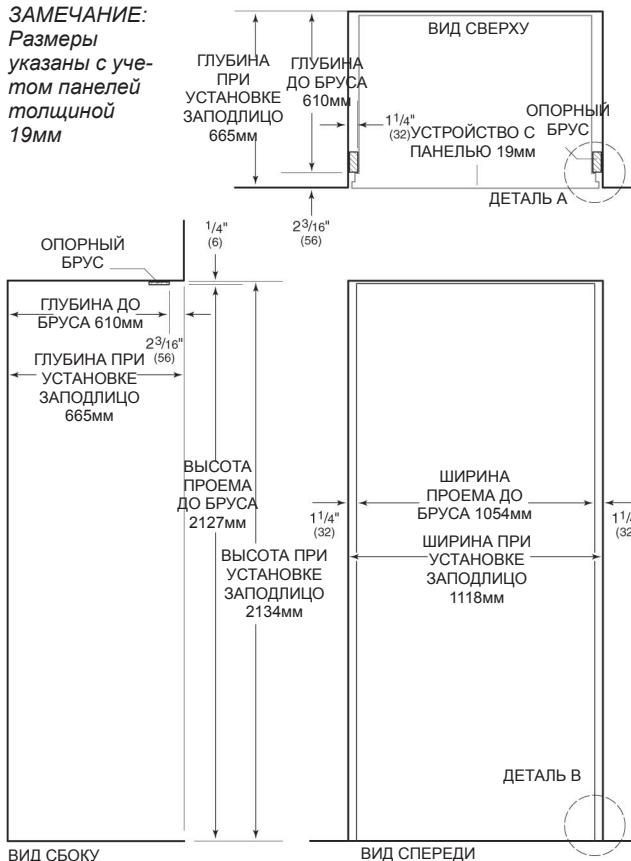
ДЕТАЛЬ А
