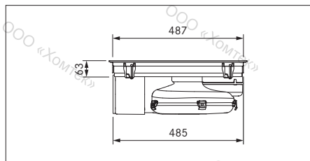
рис. 3.12 PURU Размеры устройства Вид сбоку
