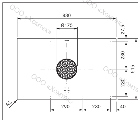
рис. 3.4 Размеры устройства PUXU Вид сверху
