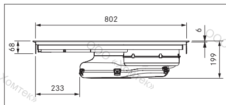
рис. 3.2 Размеры устройства PUXA Вид спереди
