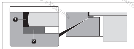
рис. 6.18 Использование уплотнительной ленты при монтаже заподлицо
