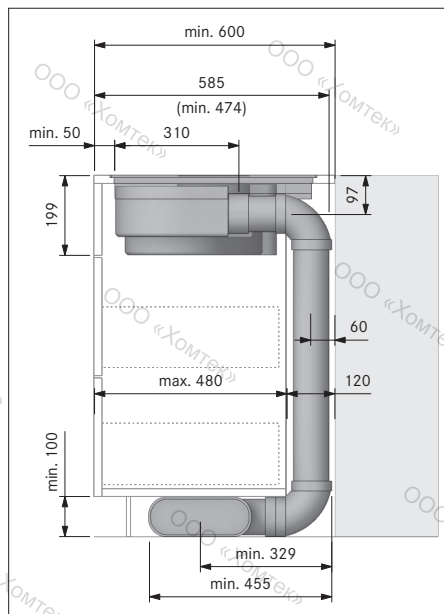
рис. 6.16 Монтажные размеры при установке вытяжной вентиляции, глубина столешницы 600 мм
