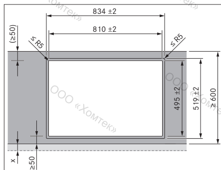
рис. 6.8 Размеры выреза для монтажа заподлицо
