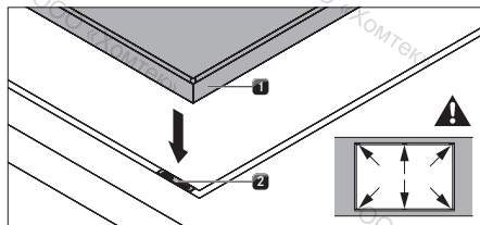
рис. 6.34 Пластины для выравнивания по высоте
