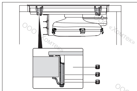
рис. 6.36 Крепление варочной панели
