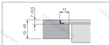
рис. 6.13 Шов для монтажа заподлицо
