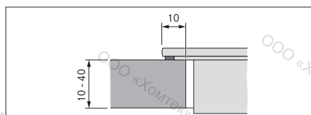
рис. 6.11 Размеры основания для навесного монтажа
