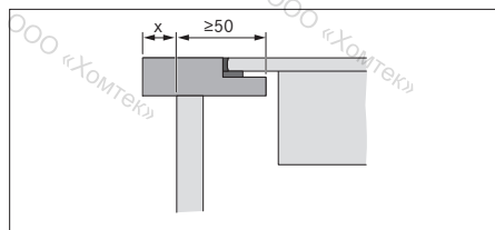
рис. 6.7 Выступ рабочей поверхности
