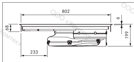
рис. 3.5 Размеры устройства PUXU Вид спереди
