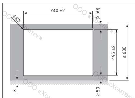
рис. 6.14 Размеры выреза для навесного монтажа
