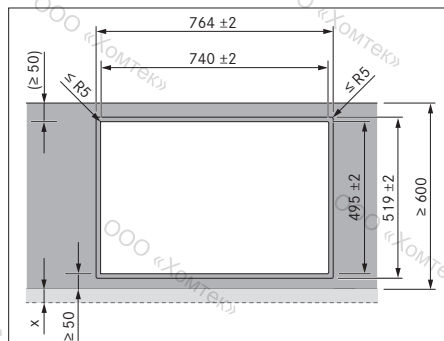
рис. 6.12 Размеры выреза для монтажа заподлицо
