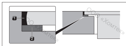
рис. 6.30 Использование уплотнительной ленты при монтаже заподлицо
