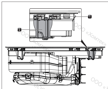
рис. 6.19 Монтаж варочной панели
