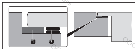
рис. 6.22 Пластины для выравнивания по высоте
