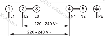
рис. 6.45 Схема подключения к двухфазной сети
