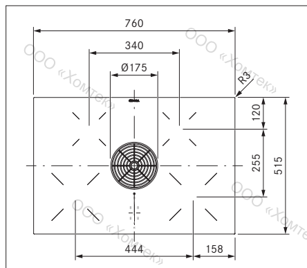
рис. 3.7 PURA Размеры устройства Вид сверху
