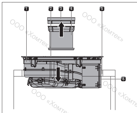
рис. 6.33 Установка варочной панели по центру
