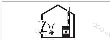
рис. 6.2 Монтаж системы отвода воздуха – правильно
