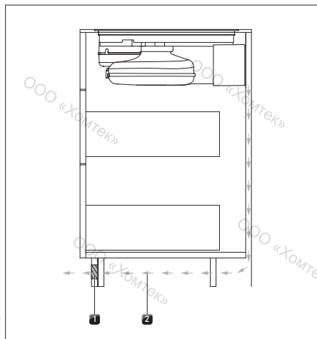
рис. 6.6 Отверстие для обратного потока в цоколе
