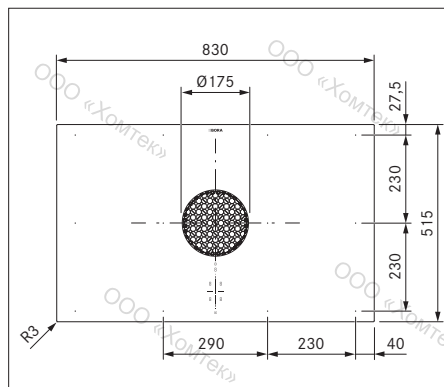
рис. 3.1 Размеры устройства PUXA Вид сверху
