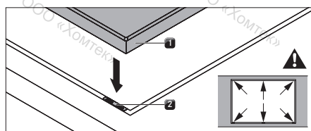
рис. 6.21 Установка пластин для выравнивания по высоте
