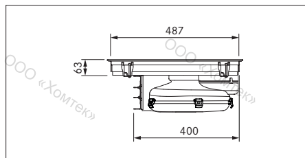
рис. 3.9 PURA Размеры устройства Вид сбоку
