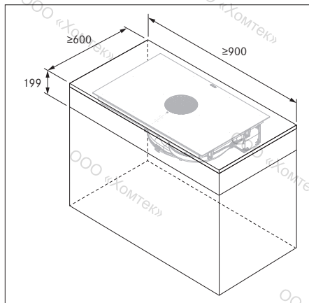
рис. 6.4 Минимальные размеры мебели X Pure
