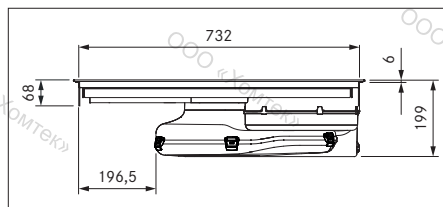
рис. 3.11 PURU Размеры устройства Вид спереди
