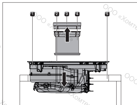
рис. 6.20 Монтаж варочной панели
