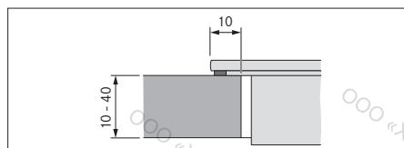
рис. 6.15 Размеры основания для навесного монтажа
