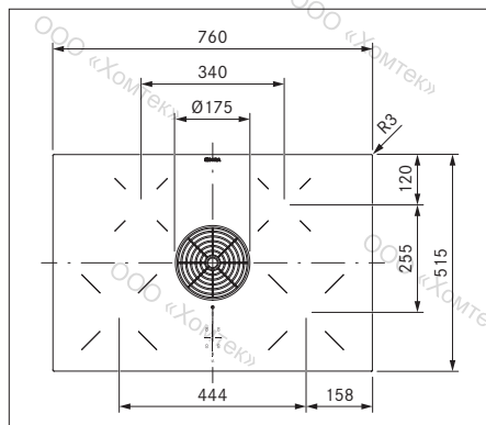
рис. 3.10 PURU Размеры устройства Вид сверху
