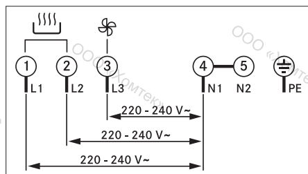
рис. 6.44 Схема подключения к трехфазной сети
