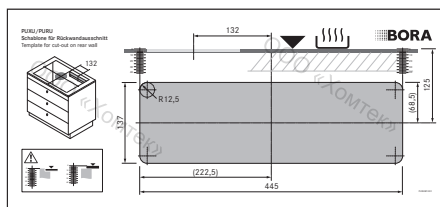
рис. 6.28 Шаблон для выреза в задней стенке
