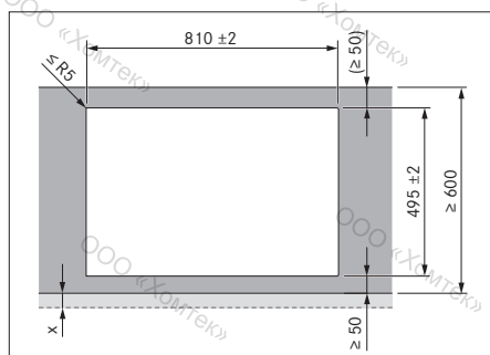
рис. 6.10 Размеры выреза для навесного монтажа
