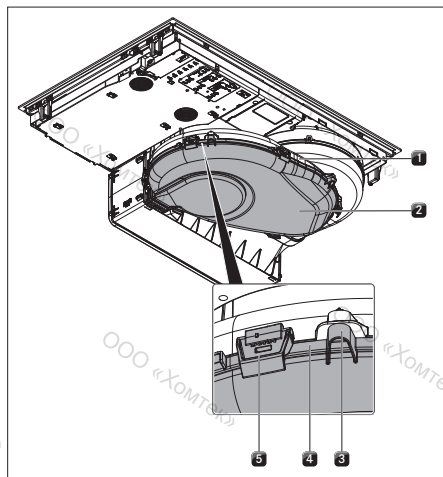
рис. 8.4 Корпус воздушного канала
