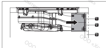
рис. 6.37 Крепление к задней стенке
