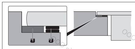
рис. 6.35 Пластины для выравнивания по высоте
