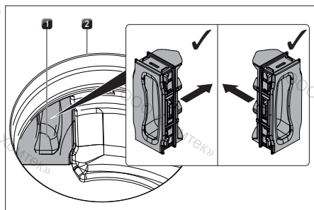
рис. 6.42 Установка откидной крышки фильтра
