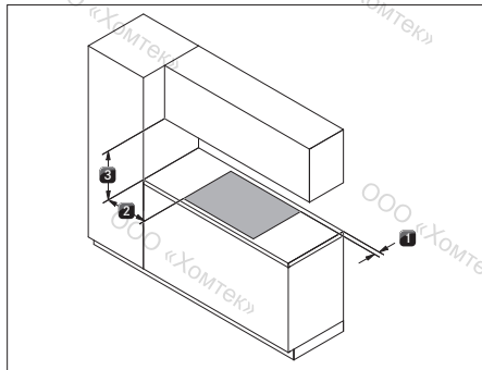
рис. 6.3 обязательные безопасные расстояния
