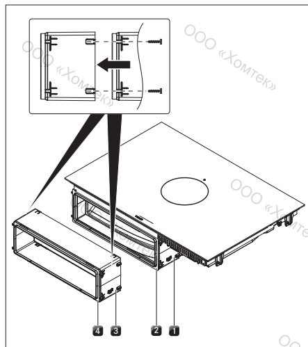
рис. 6.32 Удлинитель телескопической панели.
