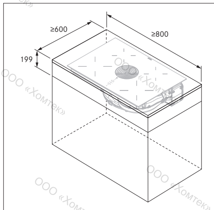
рис. 6.5 Минимальные размеры мебели Pure
