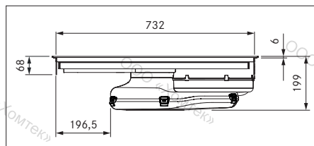
рис. 3.8 PURA Размеры устройства Вид спереди
