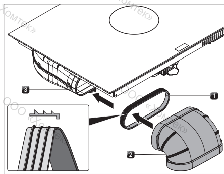
рис. 6.24 Подсоединение к системе каналов
