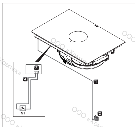
рис. 6.43 Схема подключения с опциональным модулем Home-In
