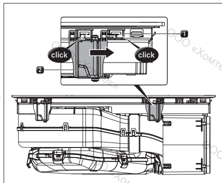
рис. 6.31 Монтаж варочной панели
