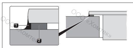
рис. 6.29 Навесной монтаж с использованием уплотнительной ленты
