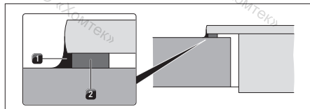
рис. 6.17 Навесной монтаж с использованием уплотнительной ленты
