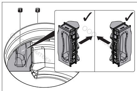
рис. 8.11 Установка откидной крышки фильтра
