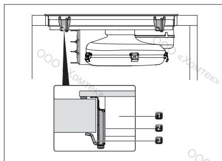
рис. 6.23 Крепление варочной панели по центру
