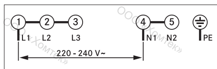
рис. 6.46 Схема подключения к однофазной сети
